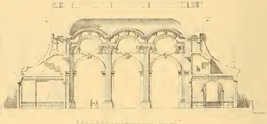
Fig. 138. Sächsisches Palais zu Warschau. Ehemaliger Gartenfaal Längschnitt.
